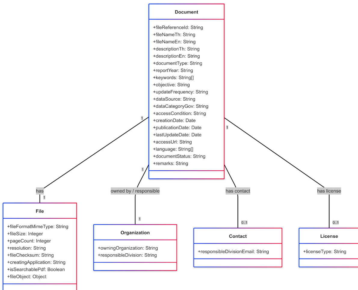
รูปที่ 1 แผนผังคลาส
