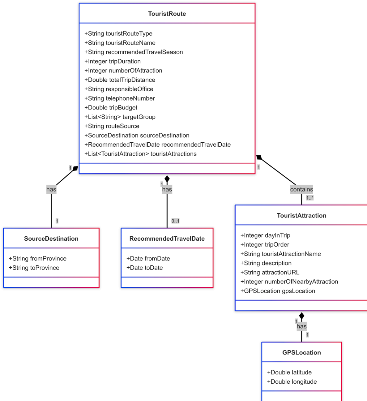
รูปที่ 1 แผนผังคลาส
