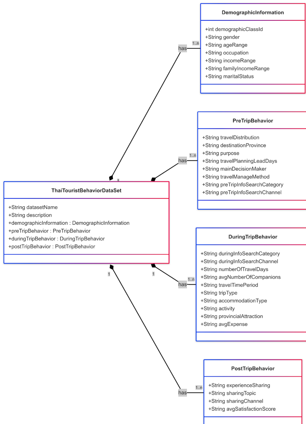
รูปที่ 1 แผนผังคลาส
